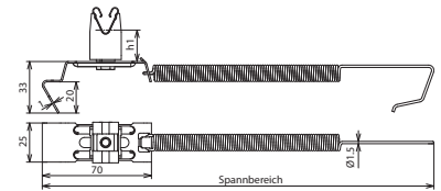
Maßbild DLH SGL 8 H20 FG180.280 V2A
