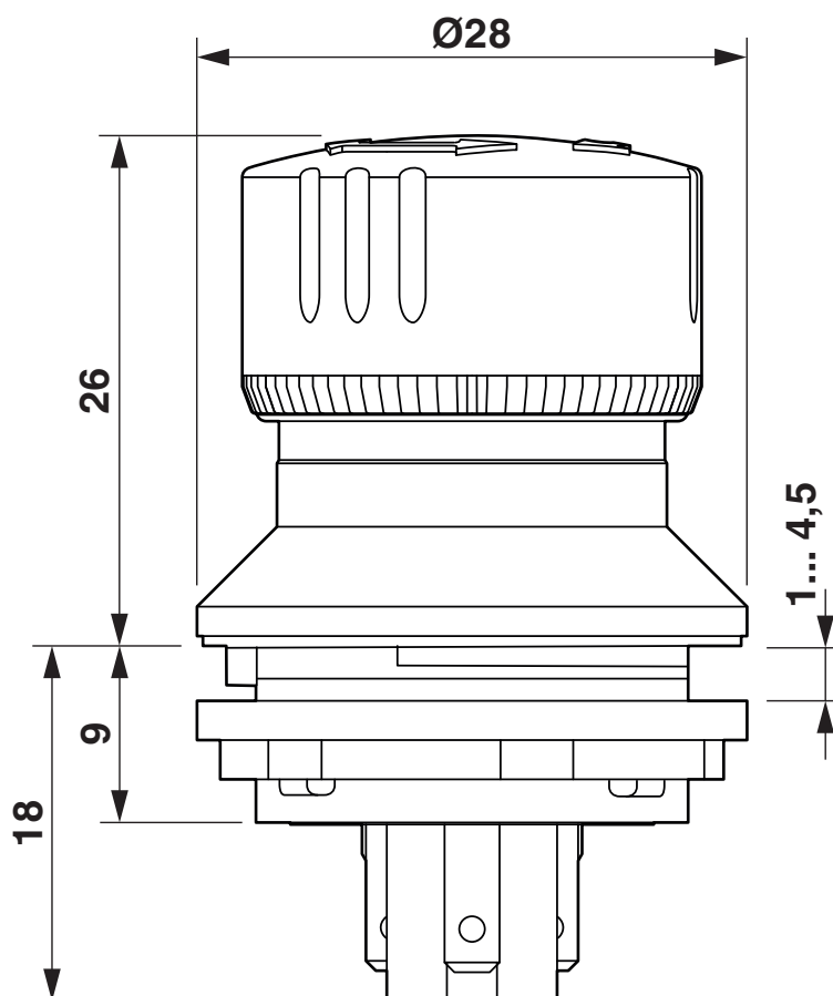
Dessin coté
