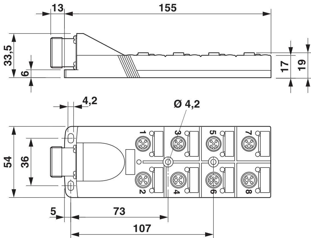
Dessin coté
