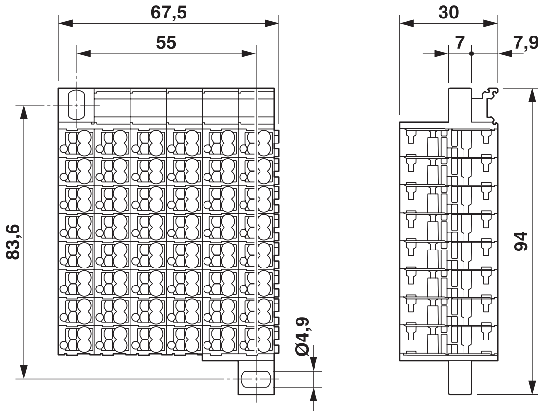
Dessin coté
