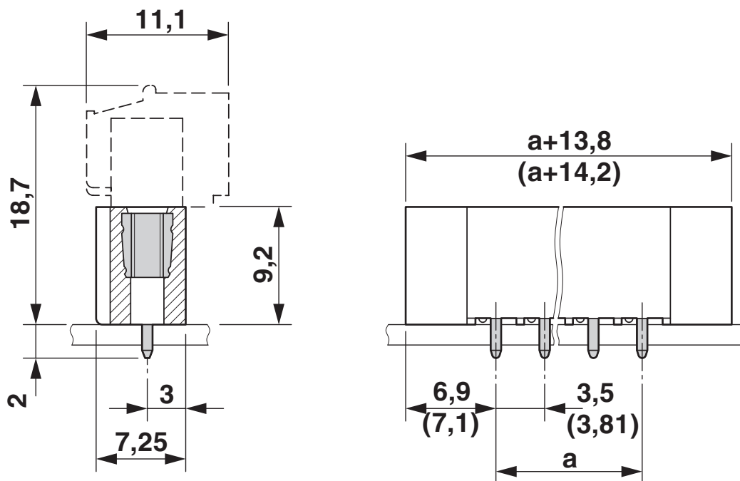
Dessin coté
