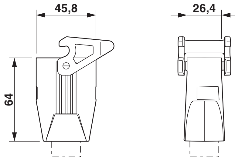
Esquema de dimensiones
