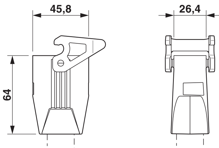
Dessin coté
