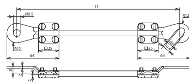
Maßbild EL10 L0.35M 1KSO 8.10 1KSG 8
