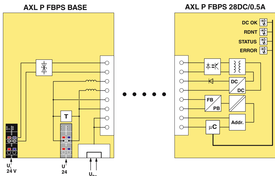
Schéma fonctionnel
