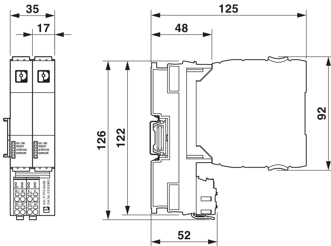
Dessin coté
