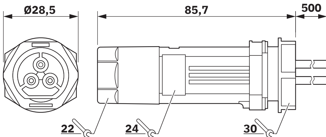
Maßzeichnung
