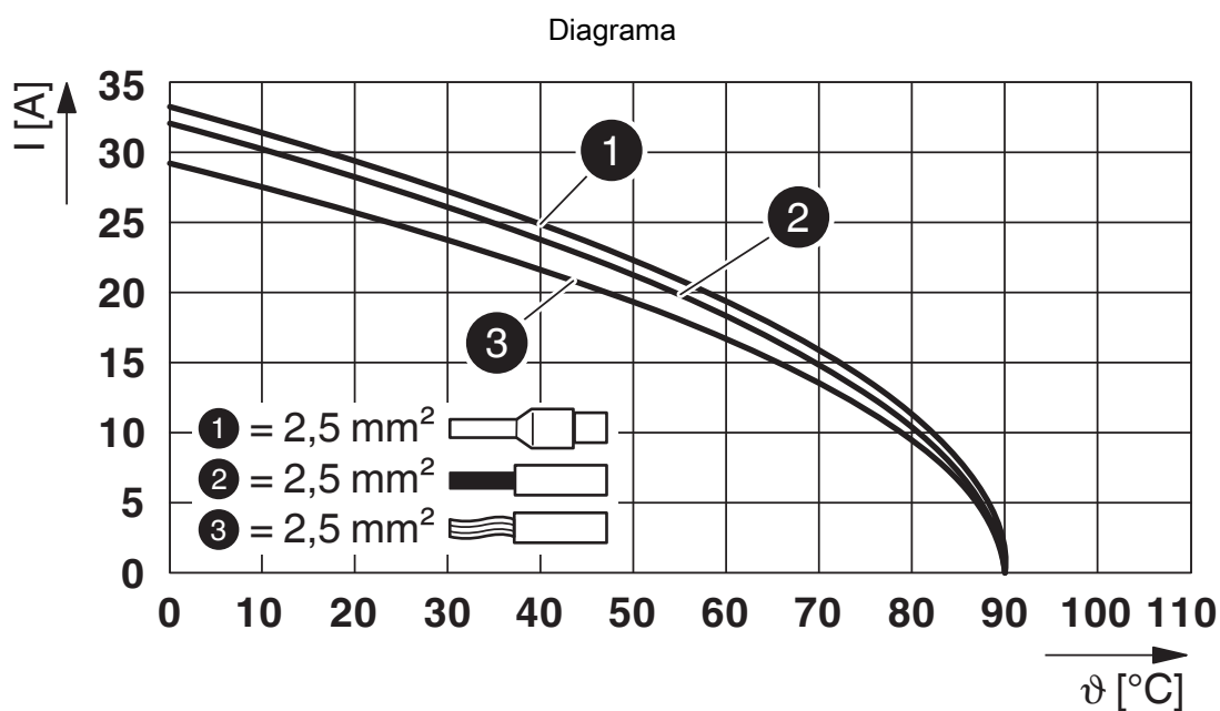
Diagrama derating para 2,5 mm 2
