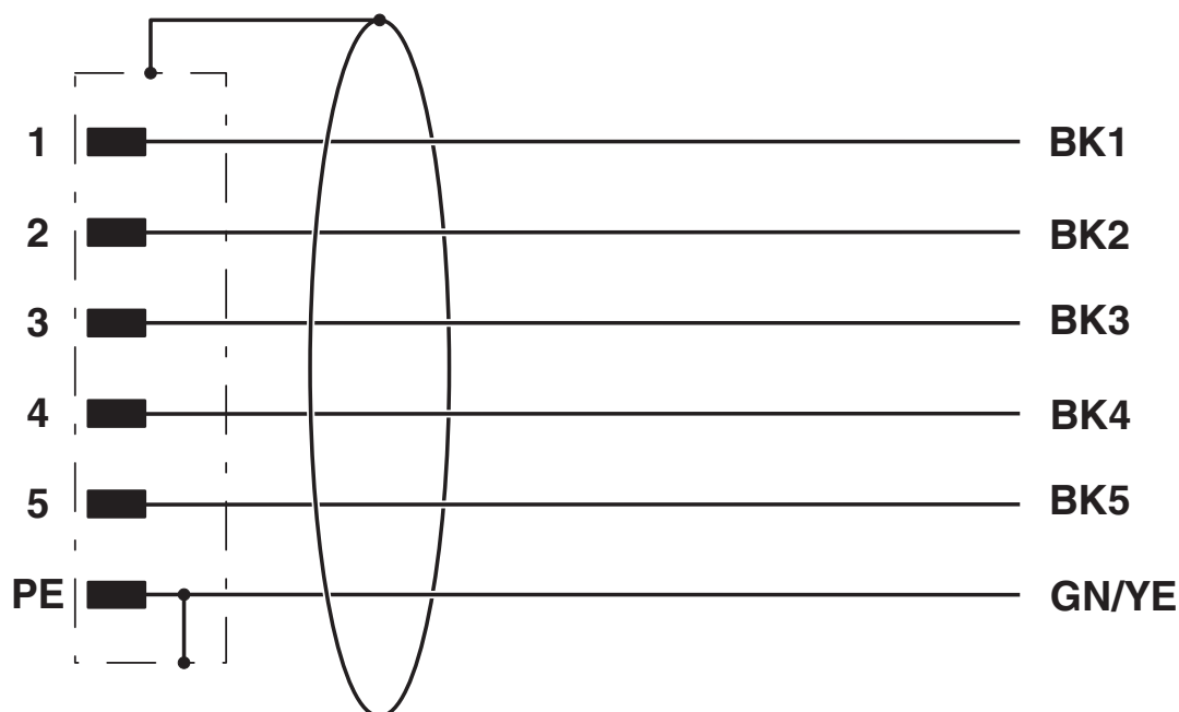
Diagrama eléctrico
