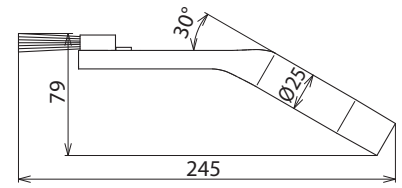
Maßbild FD 35 W P NS
