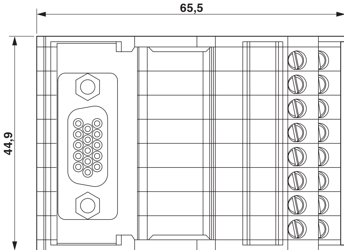
Maßzeichnung
