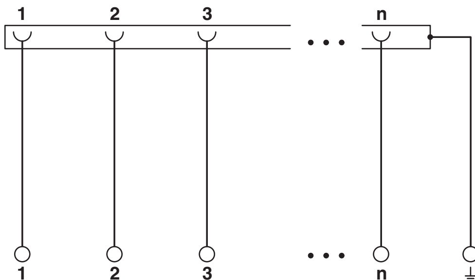
Schaltplan
