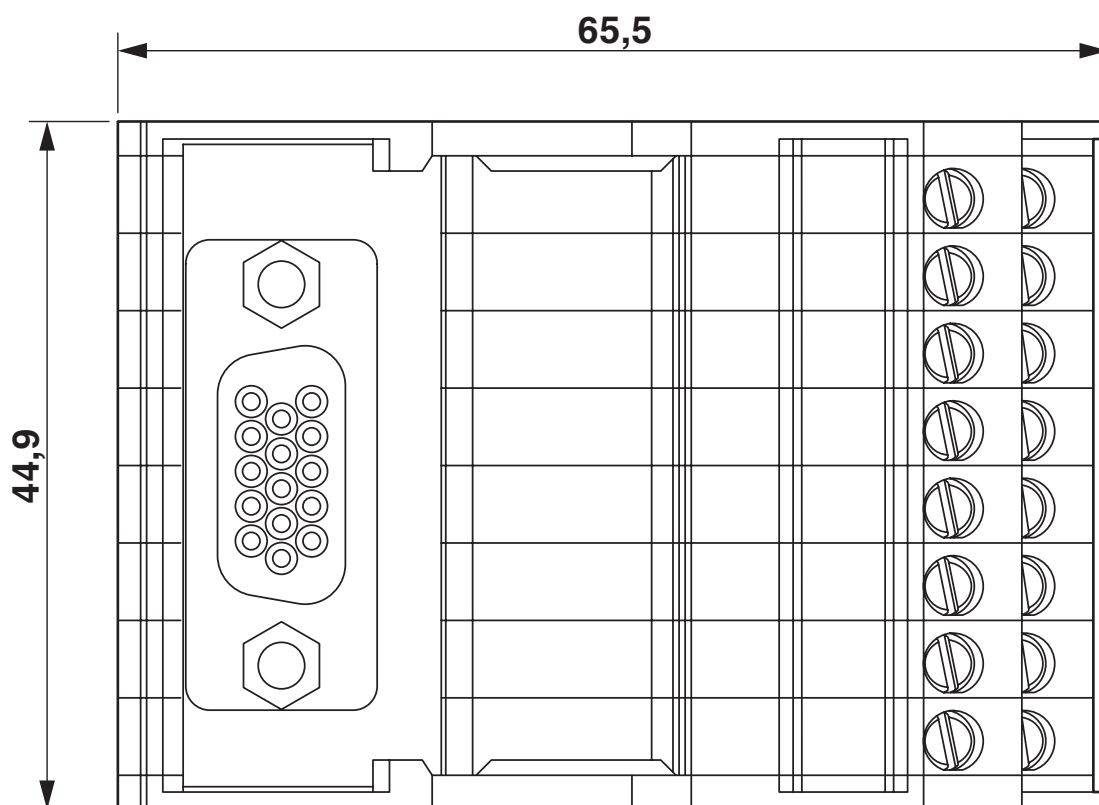
Dessin coté
