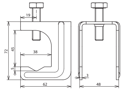
Maßbild VK 20.32 FL40 BSB STBL
