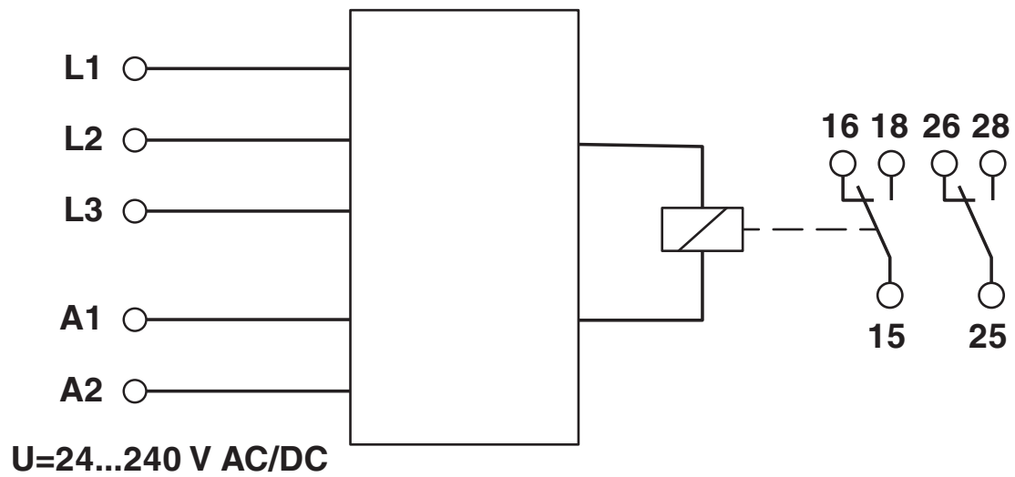
Blockschaltbild
