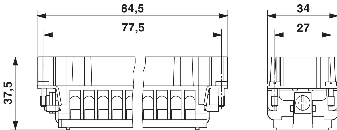
Maßzeichnung
