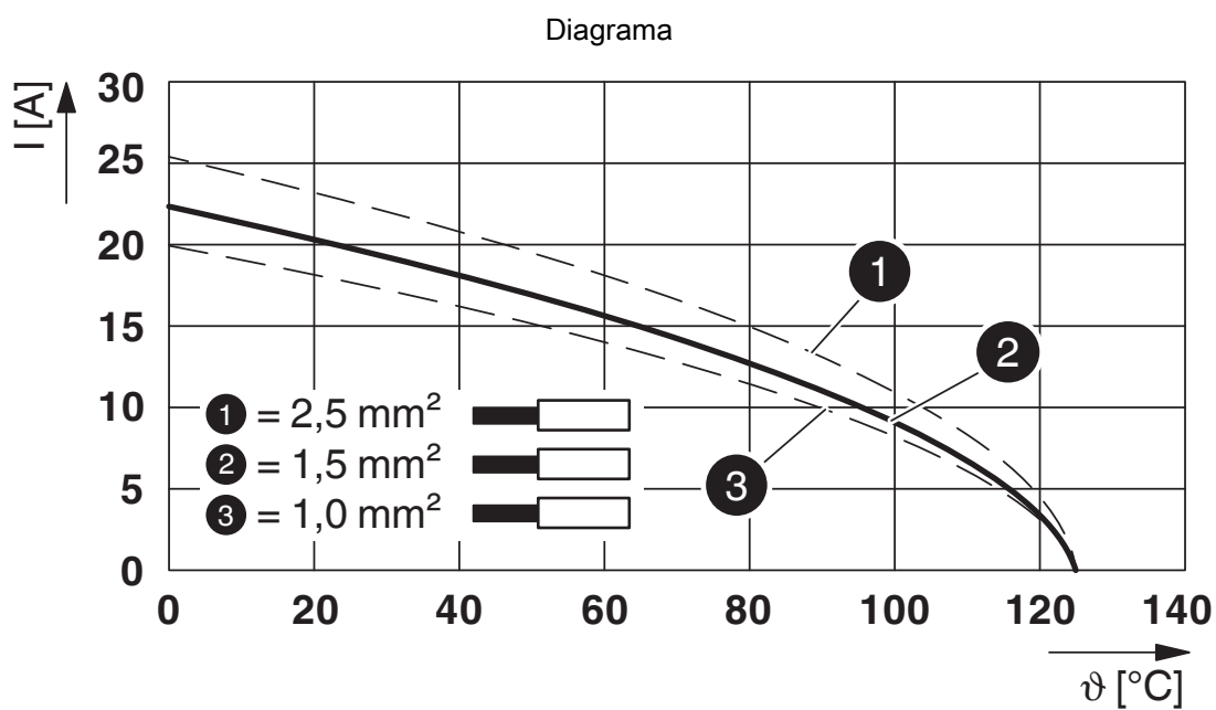
Diagrama derating para conductores rígidos
