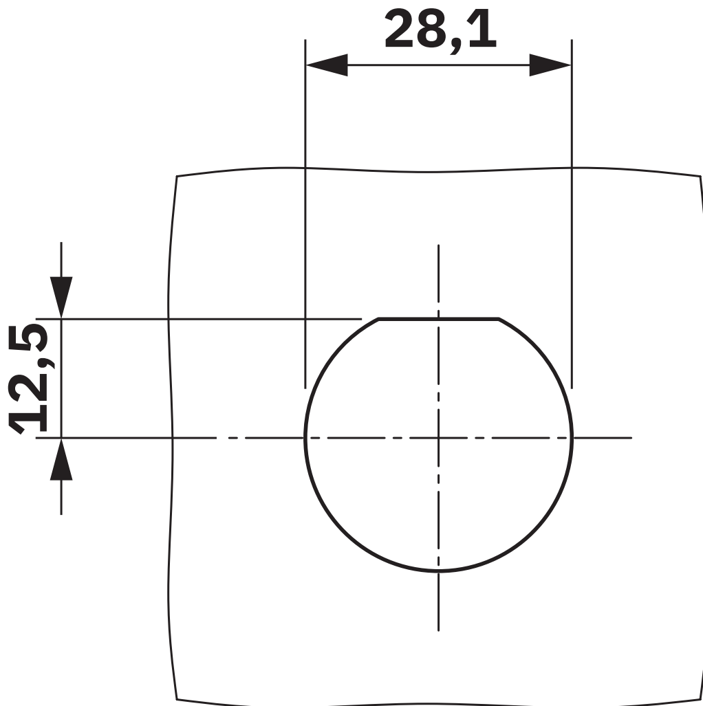
Maßzeichnung
