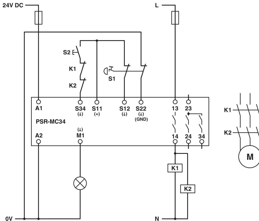
Schéma fonctionnel
