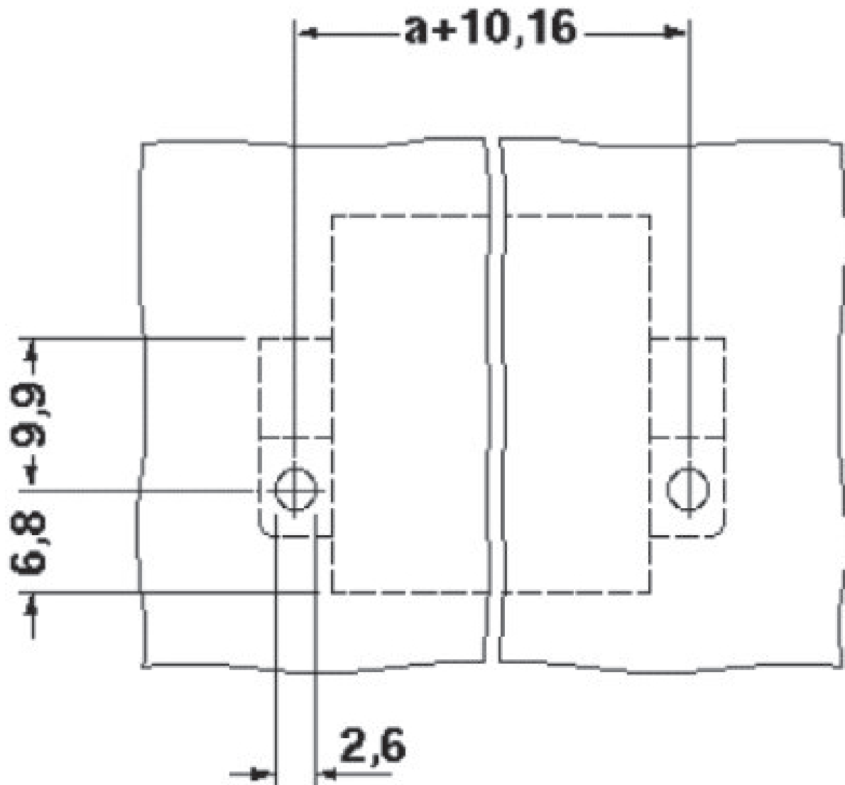
Bohrplan/Lötpadgeometrie
