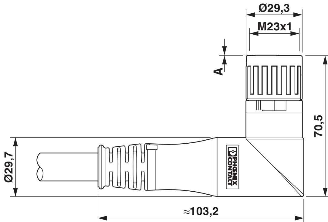
Dessin coté
