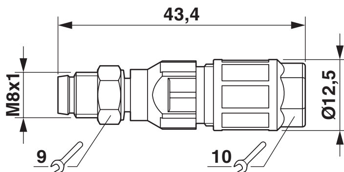
Maßzeichnung
