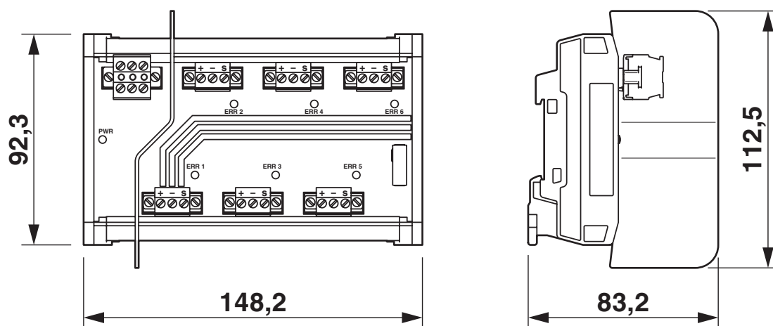
Dimensiones de FB-6SP
