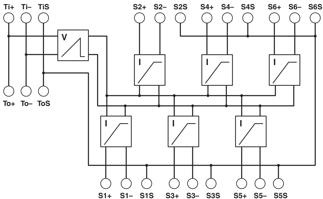
Diagrama de conexiones: FB-6SP
