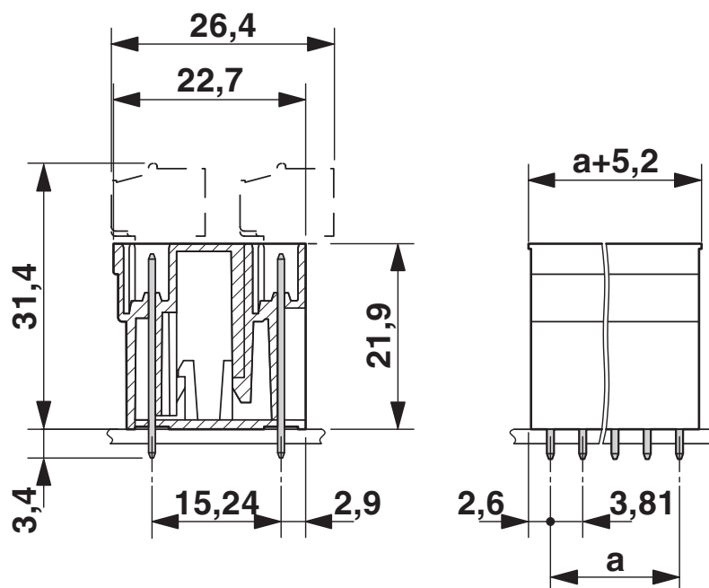
Dessin coté
