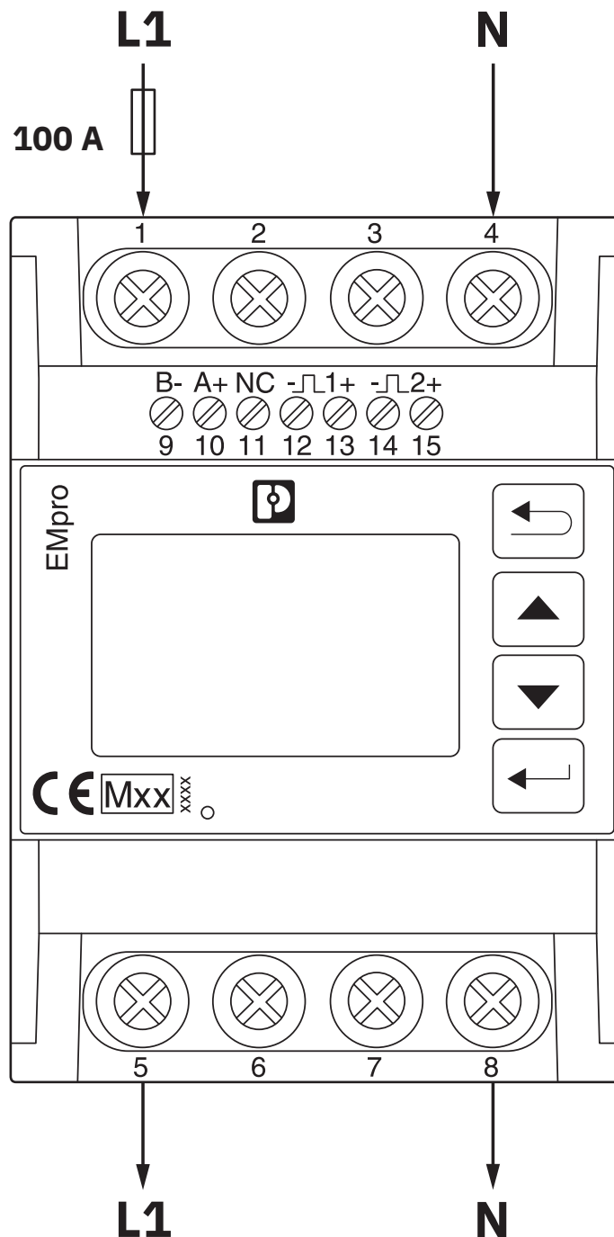
Anschlusszeichnung
