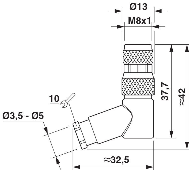
Maßzeichnung
