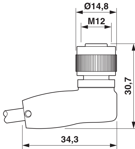
Maßzeichnung
