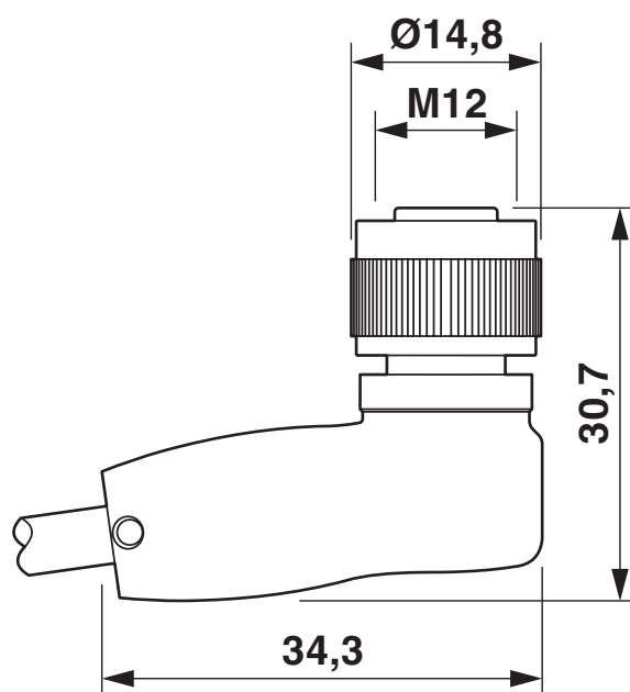
Dessin coté
