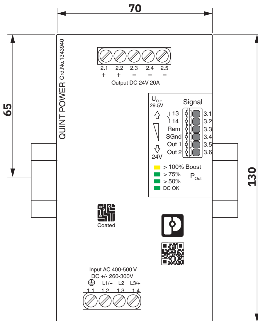
Abmessungen Vorderansicht (Maße in mm)
