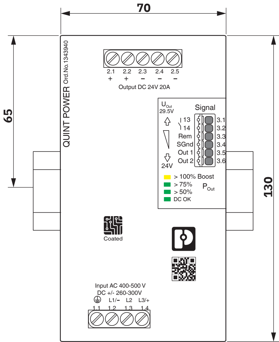
Dessin coté
