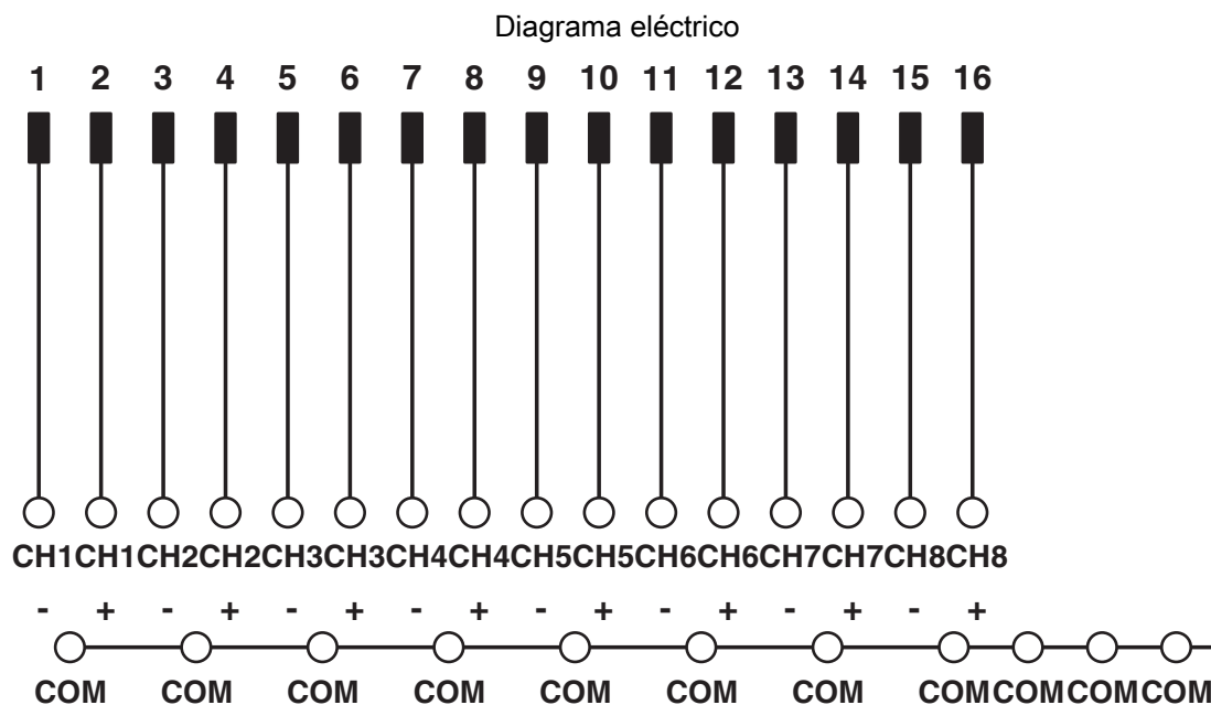
Esquema de conexiones FLKM 16/AI/DV
