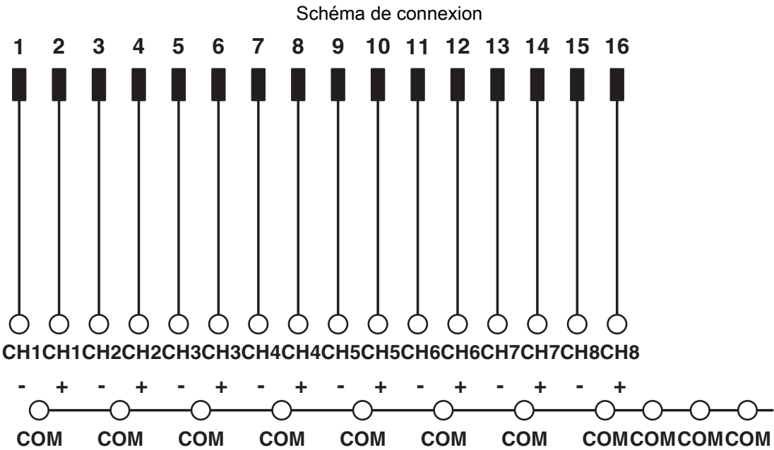
Schéma des connexions FLKM 16/AI/DV
