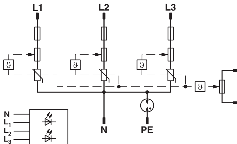
Schaltplan
