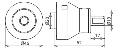
Maßbild HVI HH
