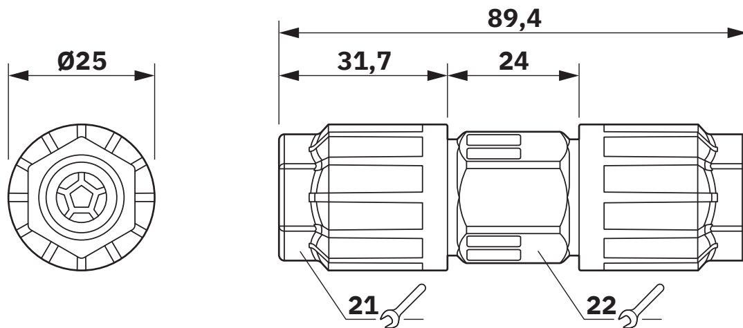
Maßzeichnung
