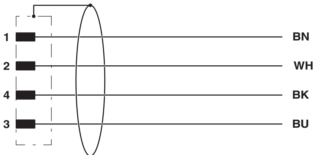
Disposition des contact des connecteurs mâles/femelles M8
