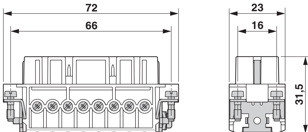
Dessin coté
