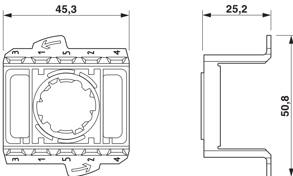
Dessin coté
