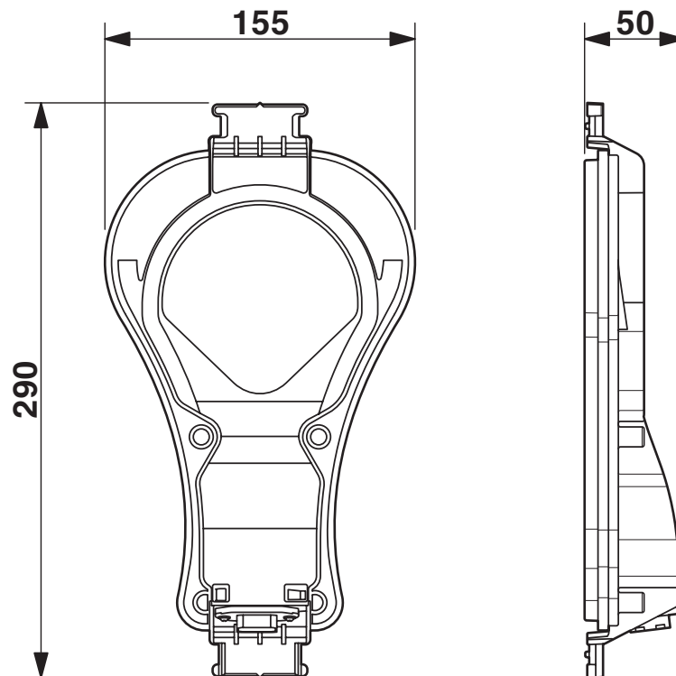
Maßzeichnung
