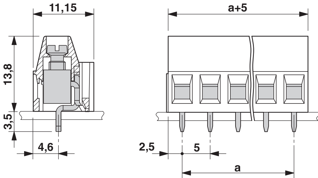
Dessin coté
