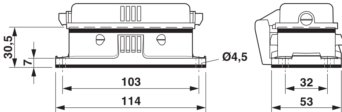
Dessin coté
