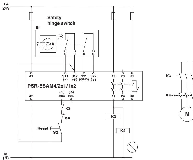
Diagrama eléctrico
