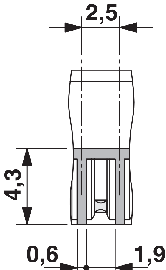
Maßzeichnung
