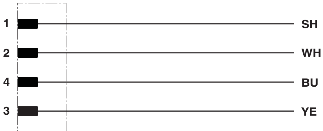
Kontaktbelegung des M12-Stecker
