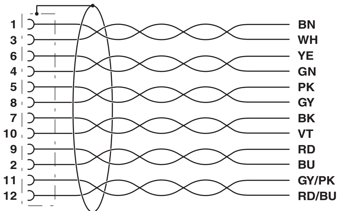
Ocupación de contactos del conector hembra M12
