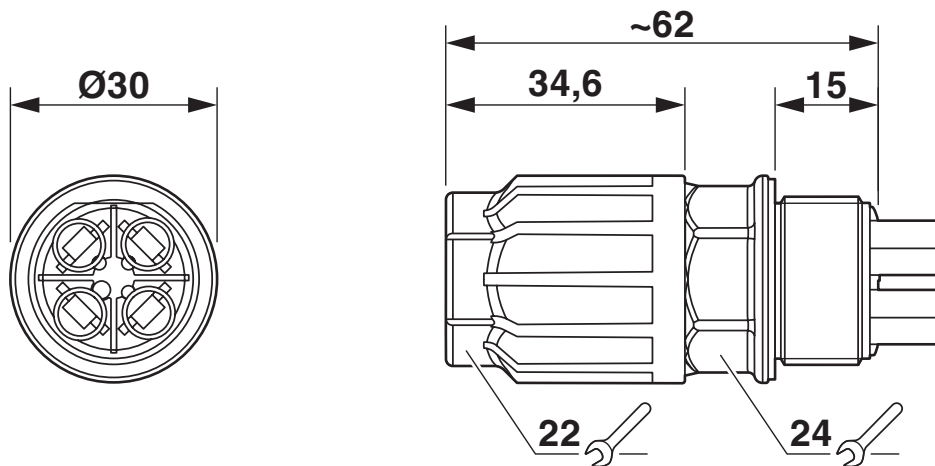
Maßzeichnung
