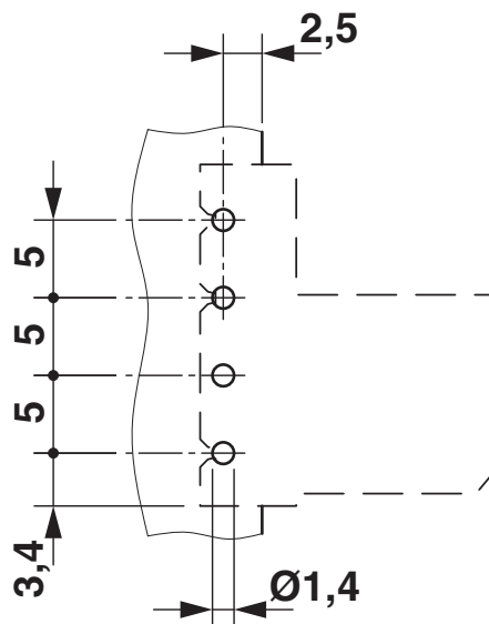
Esquema de taladros/geometría pads soldadura
