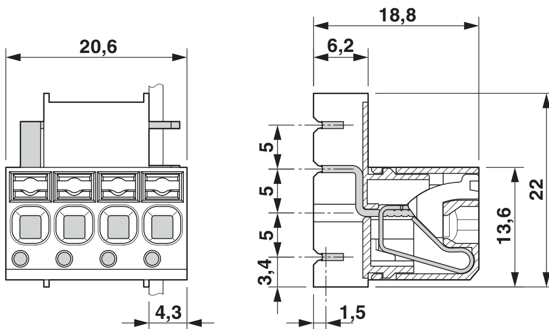
Dessin coté
